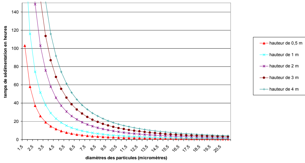
Temps de sédimentation en heures par rapport à la taille des particules
